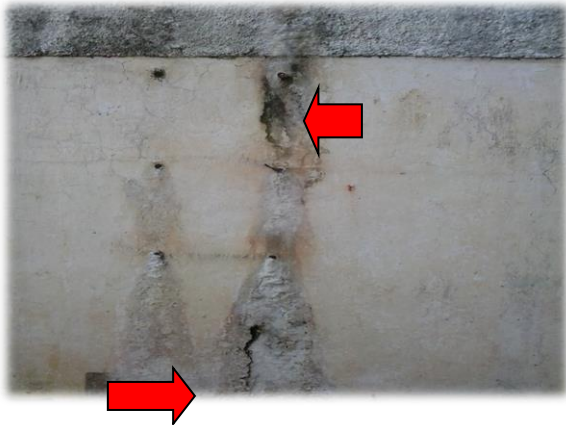
Figura 2 Percolação existente
