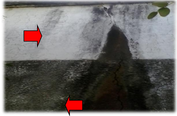
figura 3 Fissura existente
