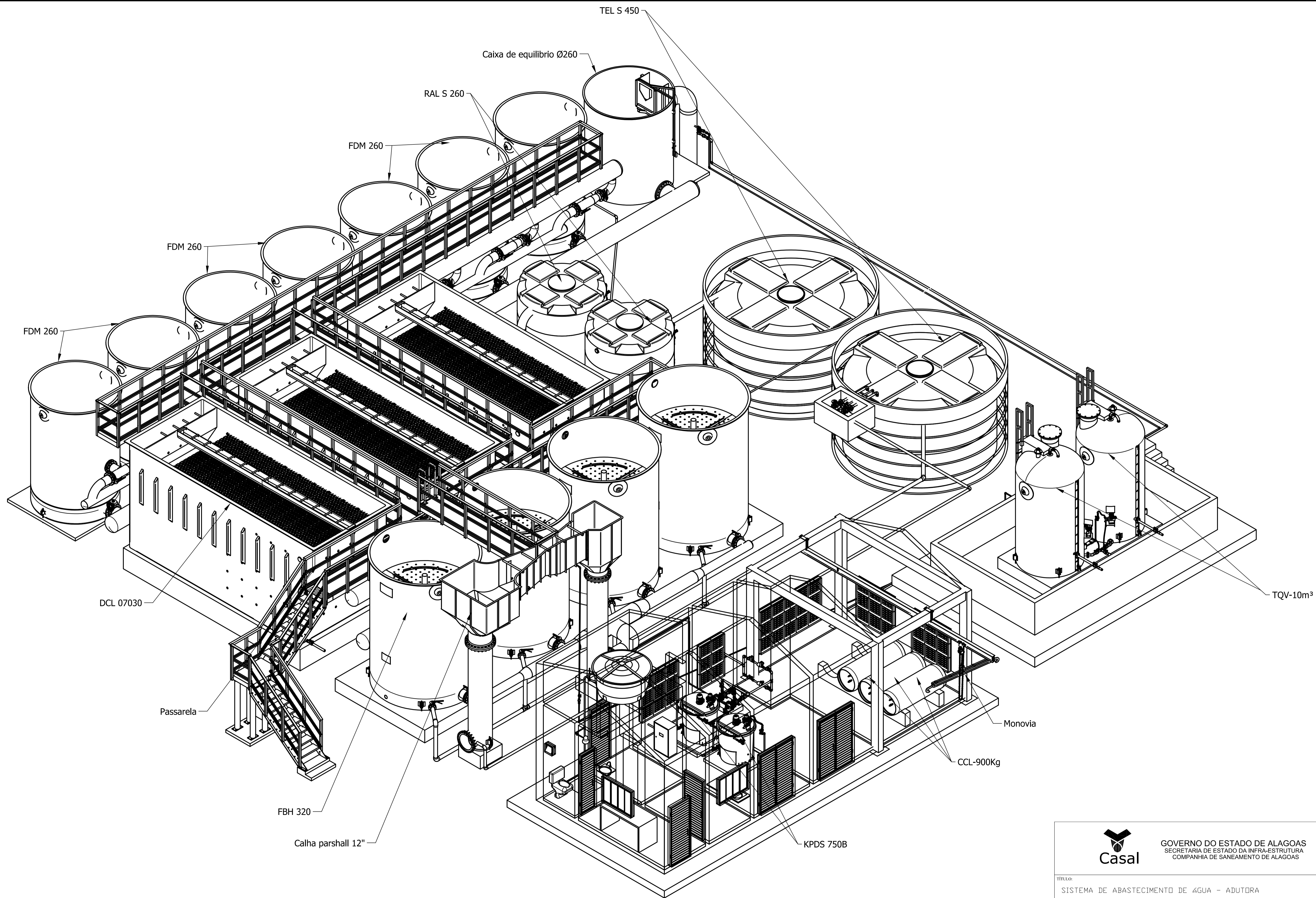
ISOMÉTRICO - ESTAÇÃO DE TRATAMENTO DE ÁGUA Esc. 1:50
