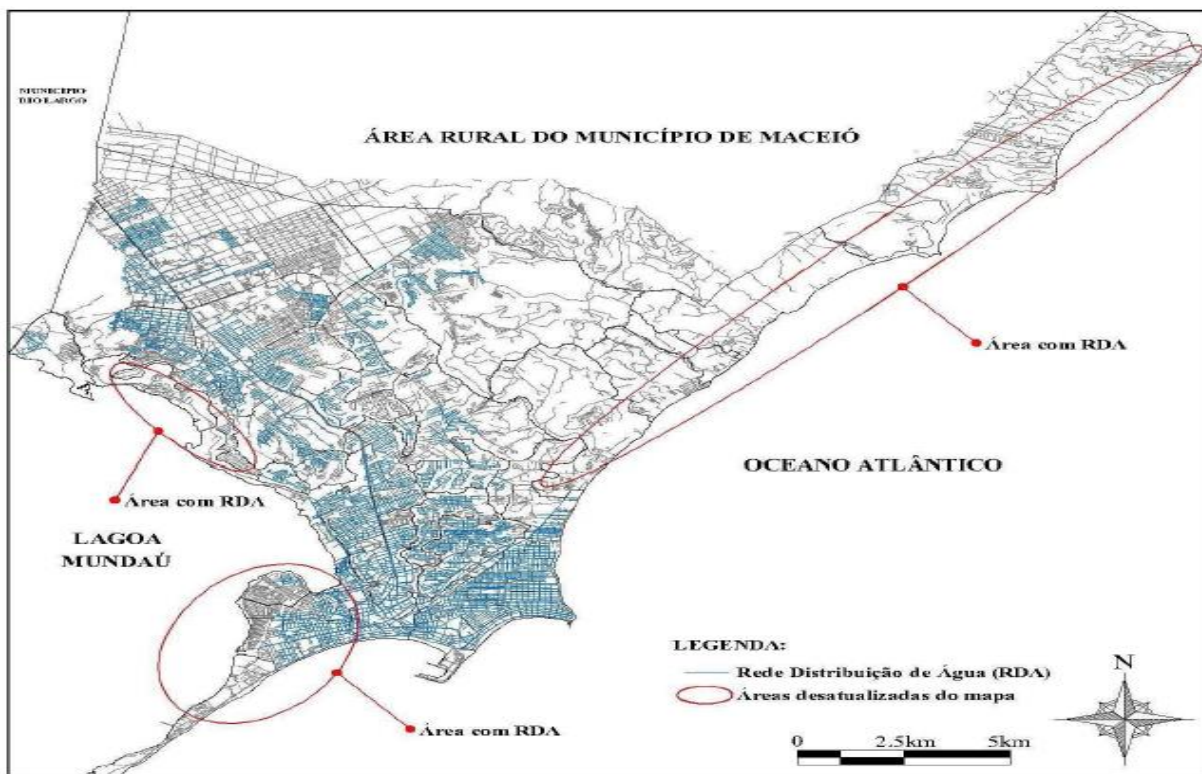
Figura 1 – Esquema de Rede de Distribuição de Maceió
