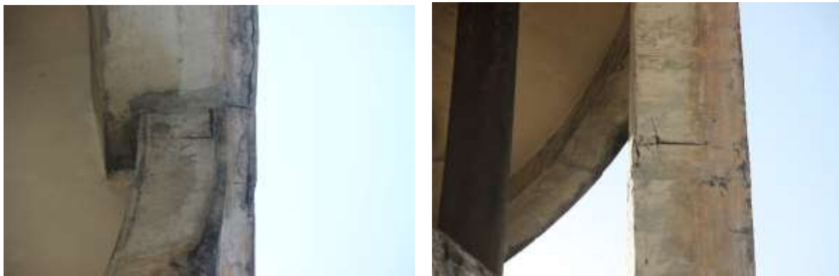
Figura 8. Deslocamento do concreto nos pilares do reservatório elevado.
