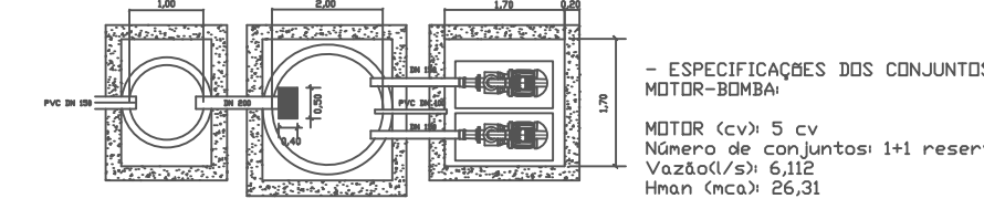
ESTAÇÃO ELEVATÓRIA Est. Livre
