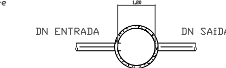
POÇO DE VISITA (PV) Est. Livre
